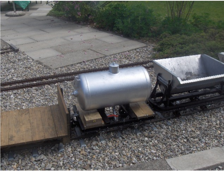
Verschiedene geplante Grubenwagen real Spurweite 7 ¼ Zoll
